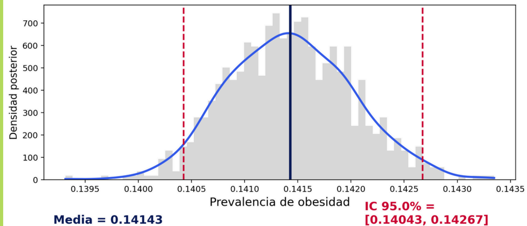
Distribución posterior de la prevalencia de obesidad (País)
