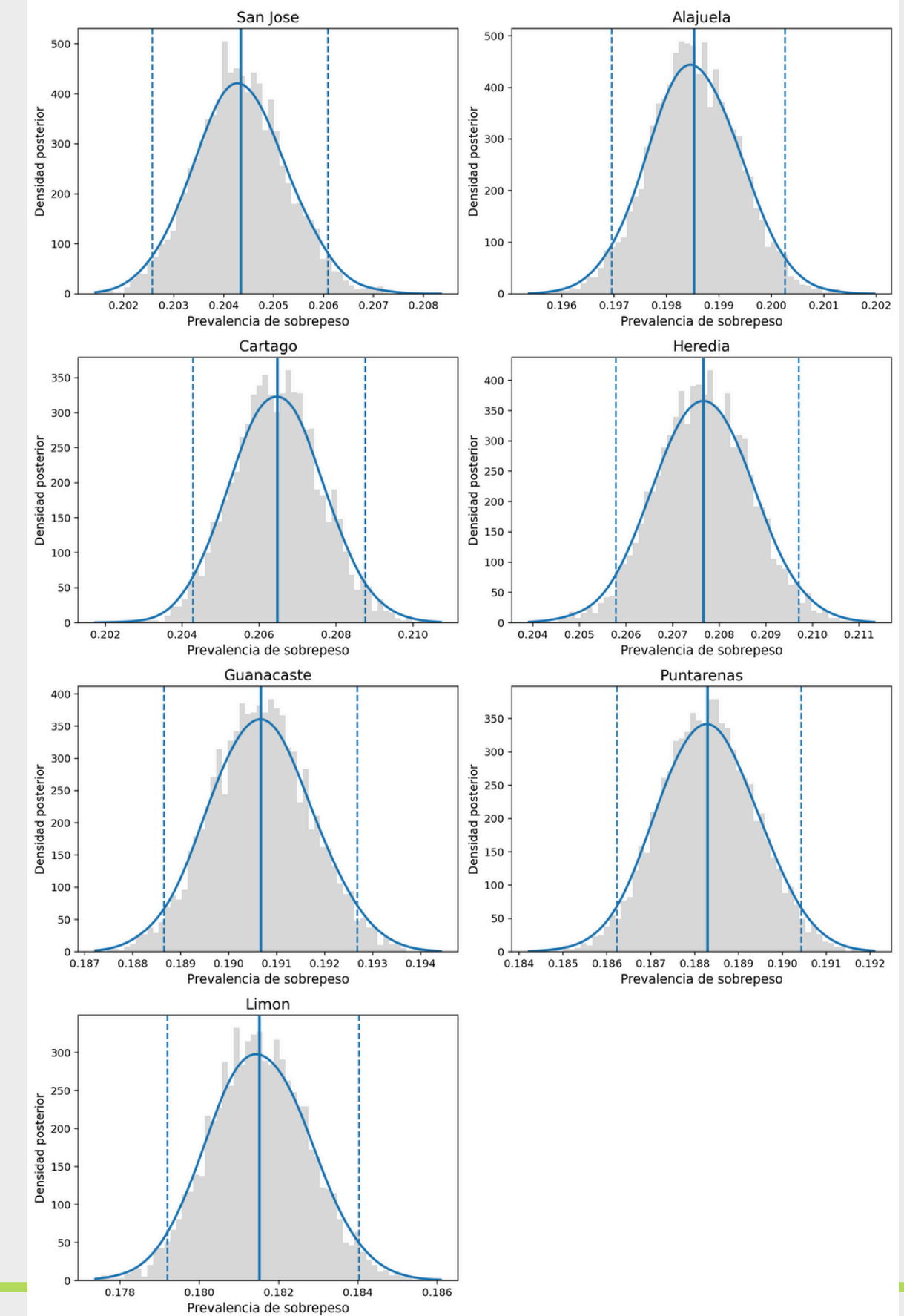
Distribuciones posteriores de la prevalencia de sobrepeso por provincia
