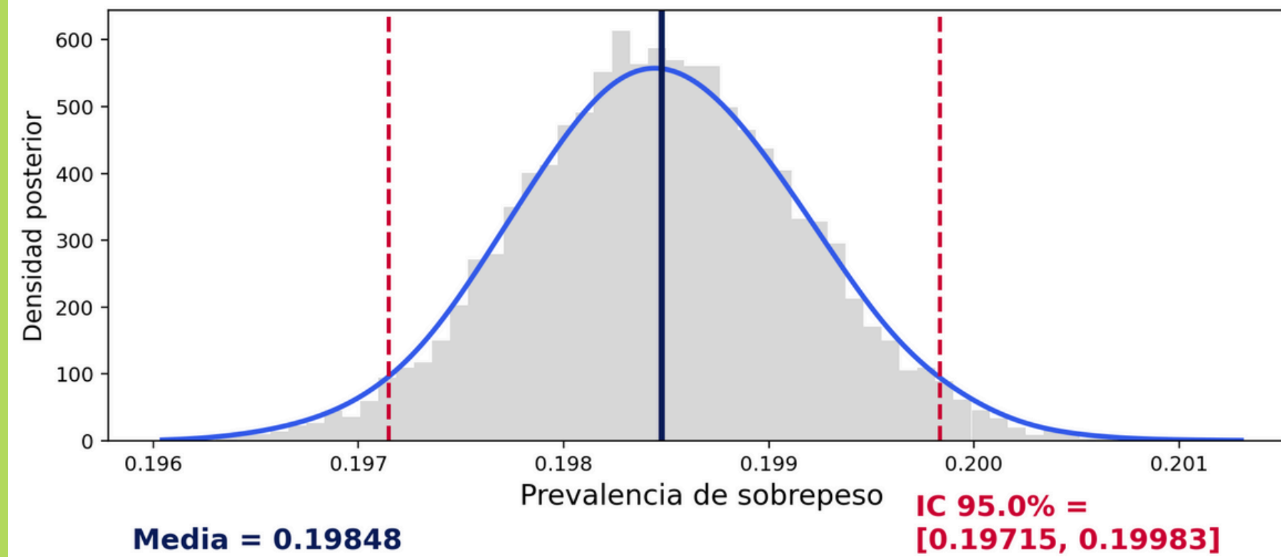
Distribución posterior de la prevalencia de sobrepeso (País)
